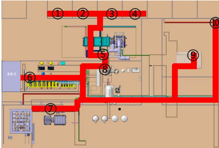
图 1 氮气管路
