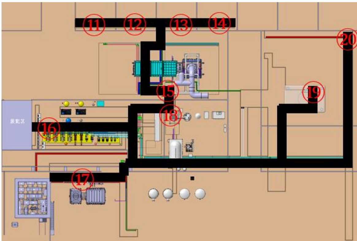
图 2 压缩空气管路
