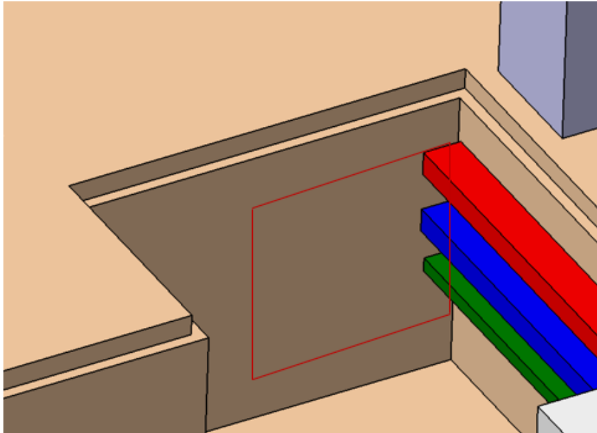
钢混墙体开洞 2m*2m 墙厚 > 0.5m 共 2 处
