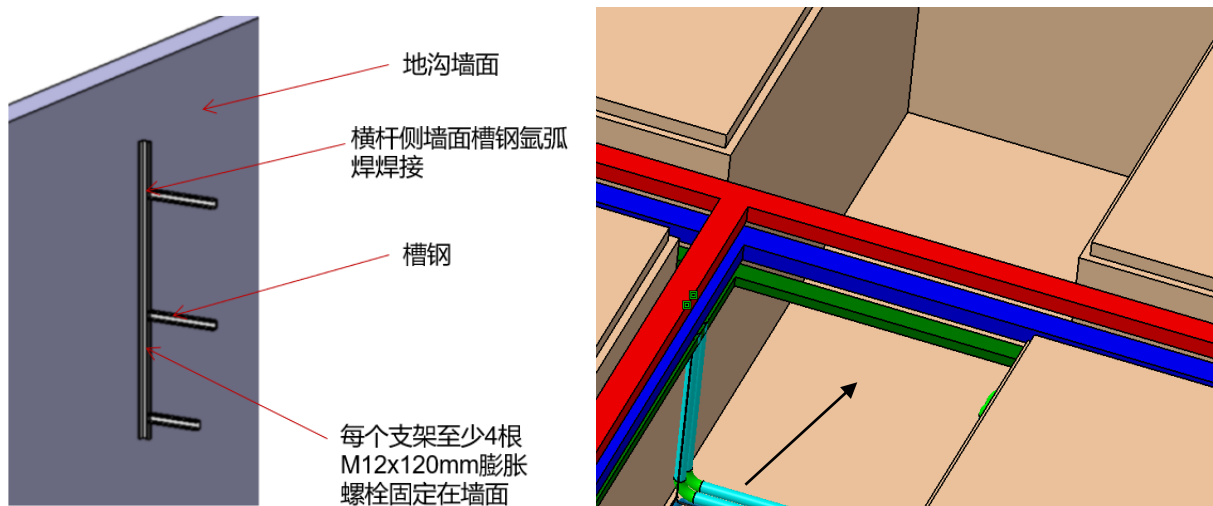
图 4 支架结构示意图
