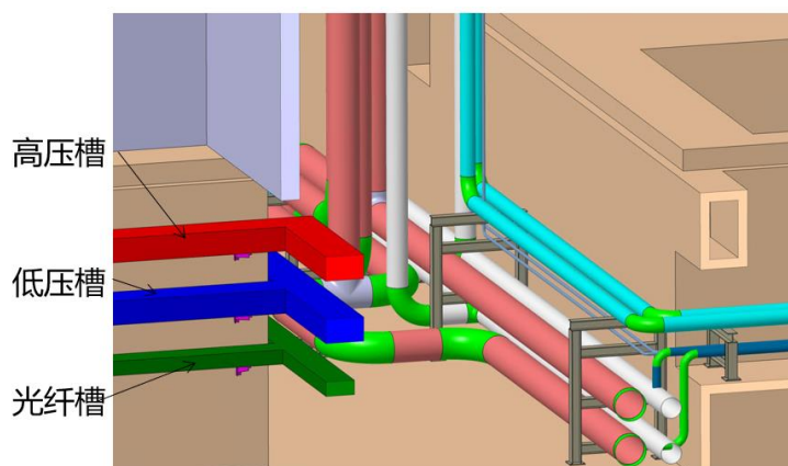
线槽排布方式示意
