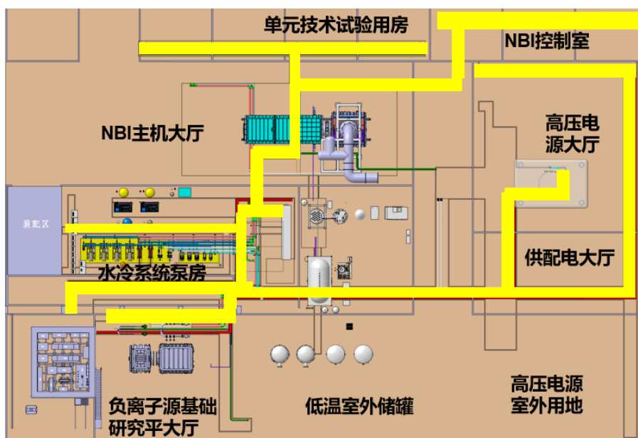
图中黄色色为光纤线槽
