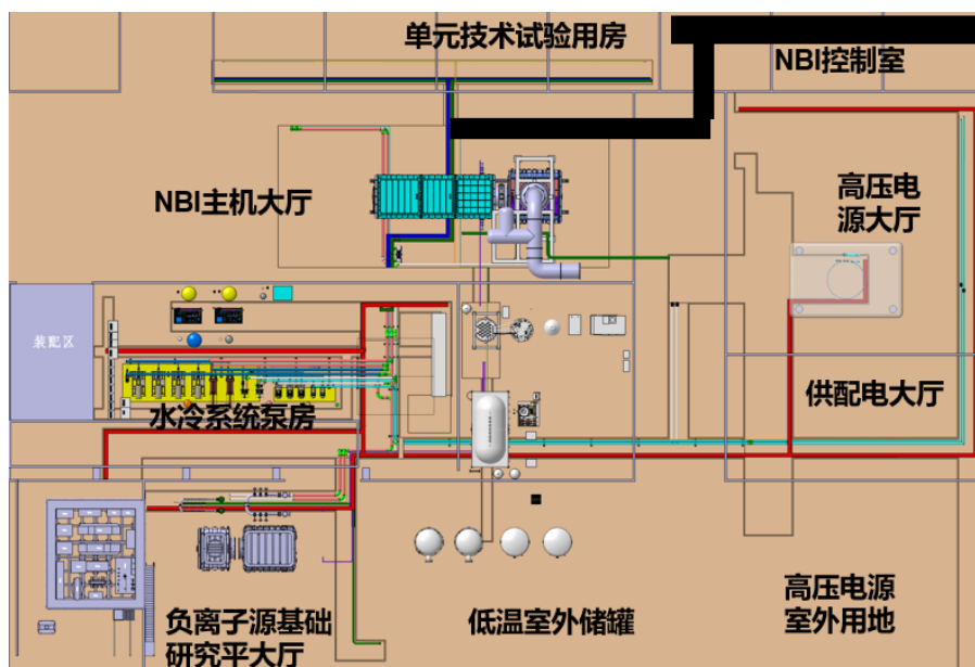
图中黑色为负二楼光纤线槽规格 100x100
