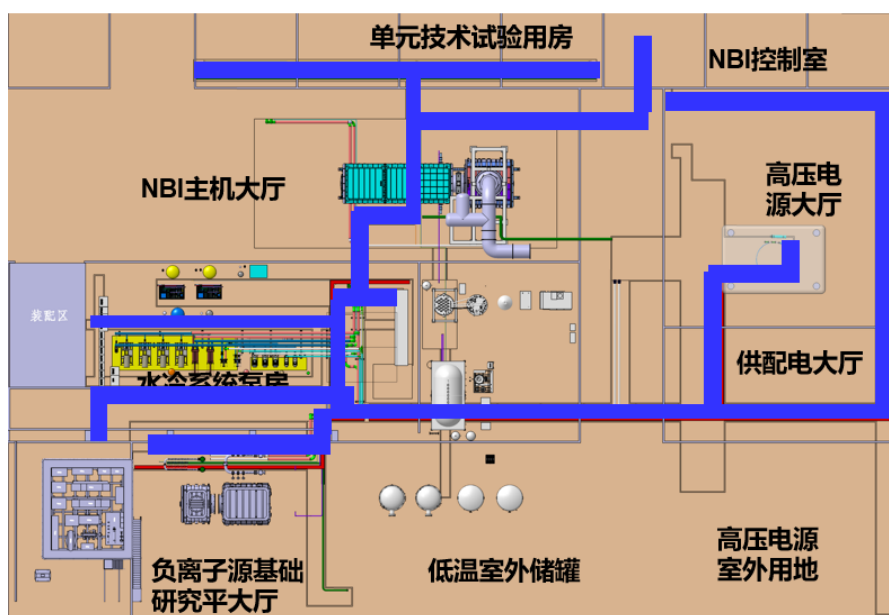
图中蓝色为低压线槽
