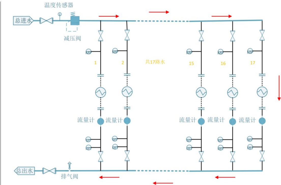
图 1. CSMC 电源水冷系统 PID 图
