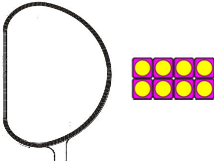
图 1 4\times 2 高场绕组及绕组截面示意图
