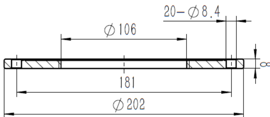
图 1、负载接口法兰盘尺寸
