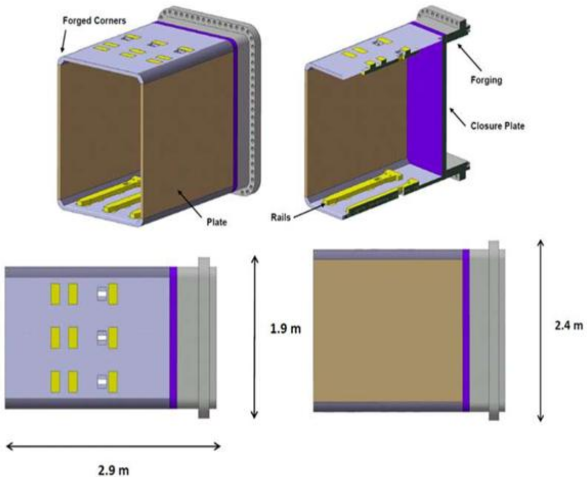
图 1 水平窗口插件结构及主要尺寸
