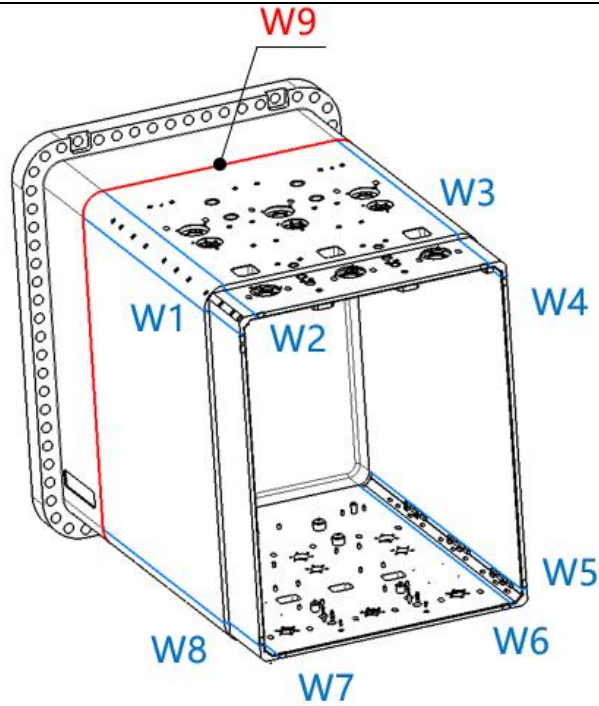
图 2 水平窗口插件焊缝分布
