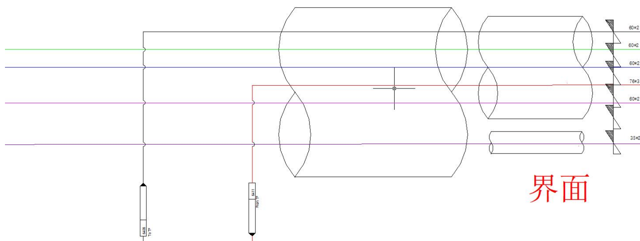
图 3.23 阀箱出口 2 低温管道（共用阀箱真空机组）
