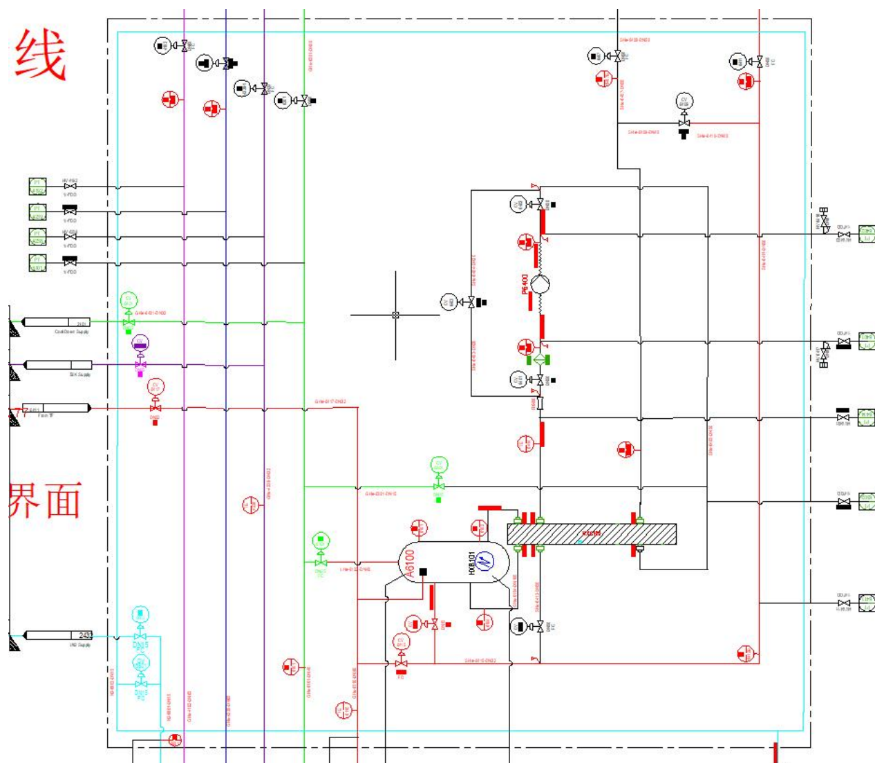
图 2. 分配系统初步流程图
