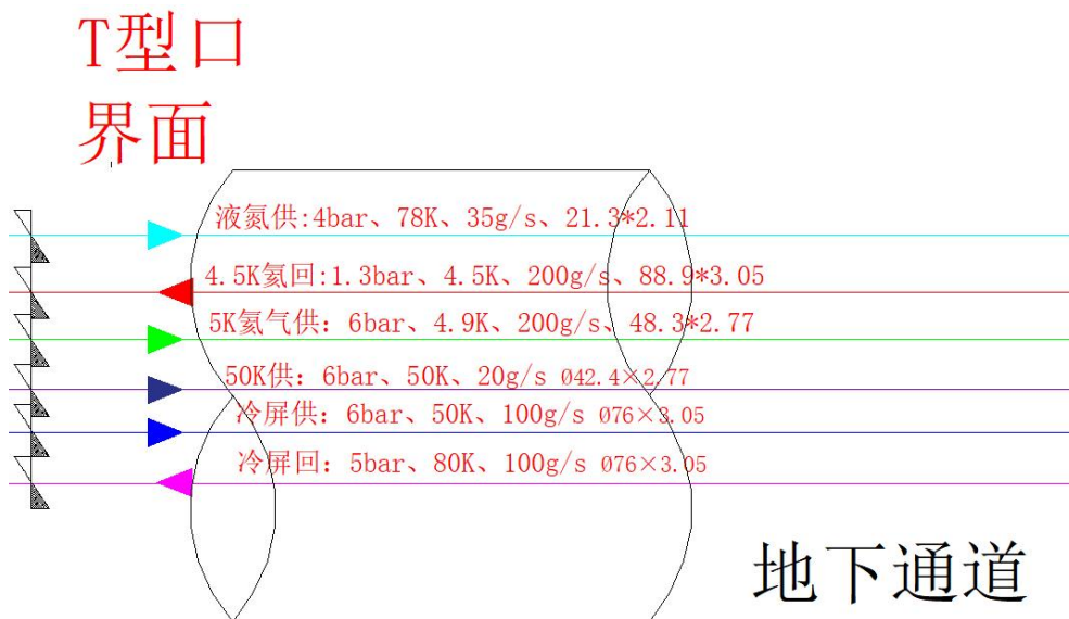
图 3.1 阀箱入口低温管道（含真空隔断及真空机组）
