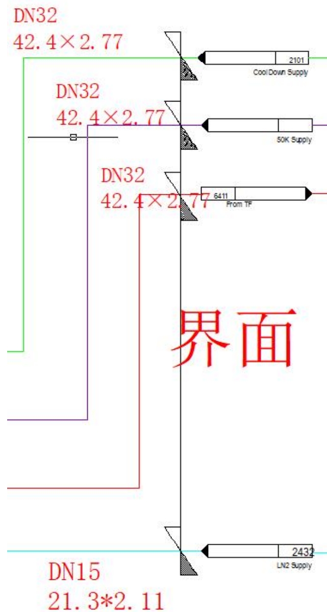
图 3.2 阀箱出口 1 真空隔断
