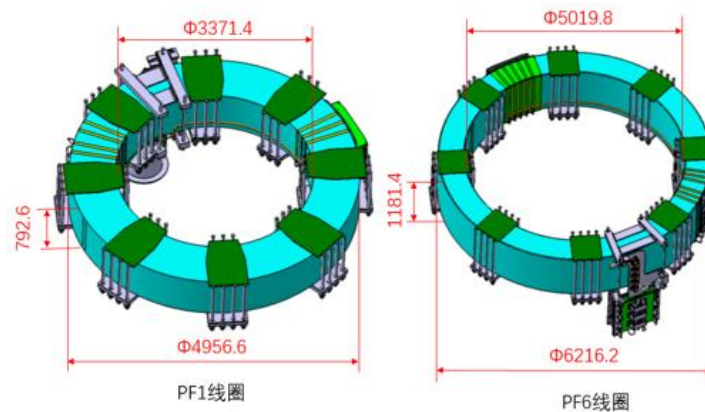
图1 BEST PF1、PF6 磁体尺寸
