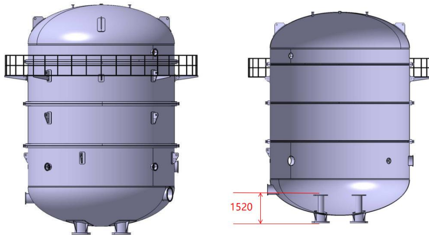
图3 CC 测试平台真空杜瓦结构尺寸
