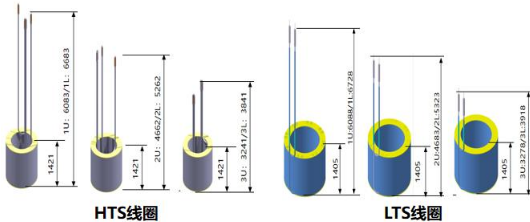
图2 BEST CS (HTS/LTS) 磁体尺寸
