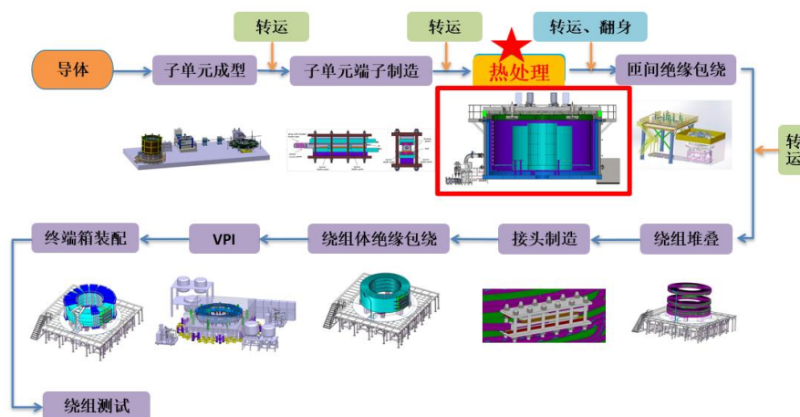
图 1 PF1/6/7 线圈制造流程图
