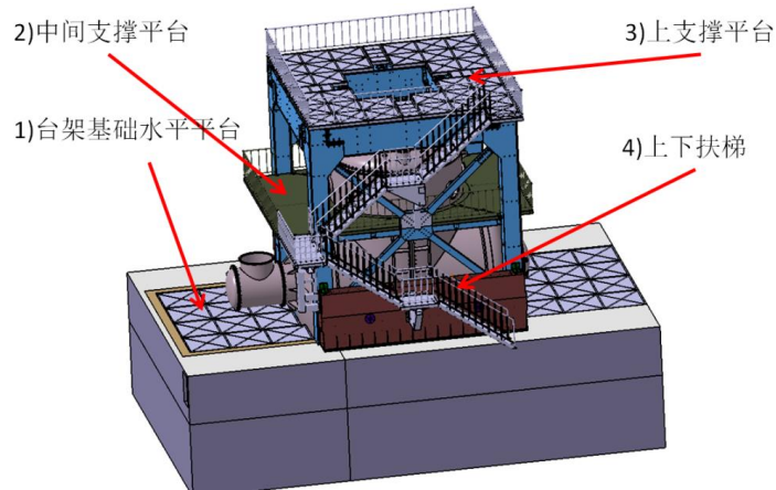
图 台架增项名称及安装位置
