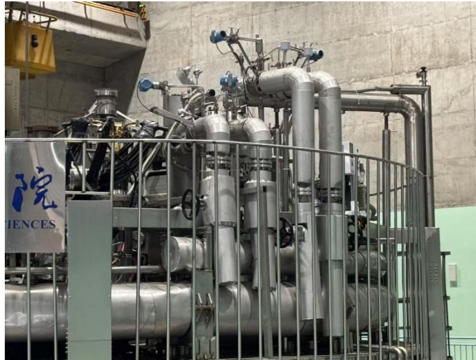
图 7 上窗口支路配置情况（上供下回）
