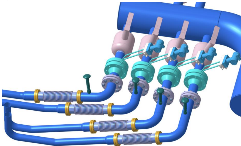
图3 下窗口供水支路配置
