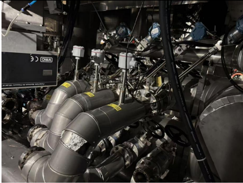
图 4 下窗口部分支路现场配置（上供下回）
