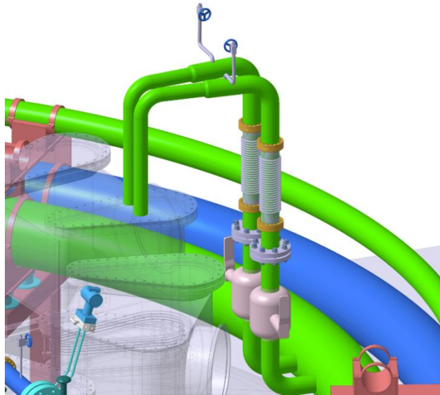
图 5 上窗口供水支路配置
