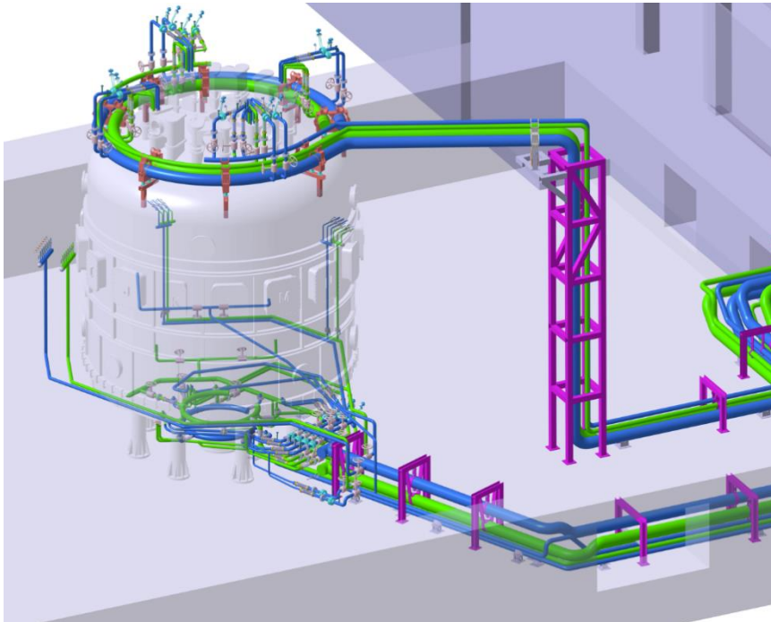
图 1 EAST 主机厅高温高压管网布局图
