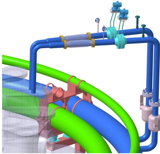
图 6 上窗口回水支路配置
