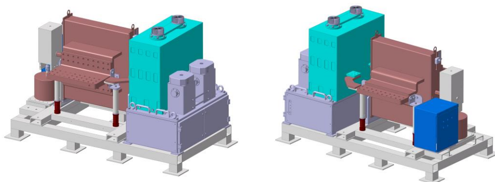
图 1 失超保护主开关模型
