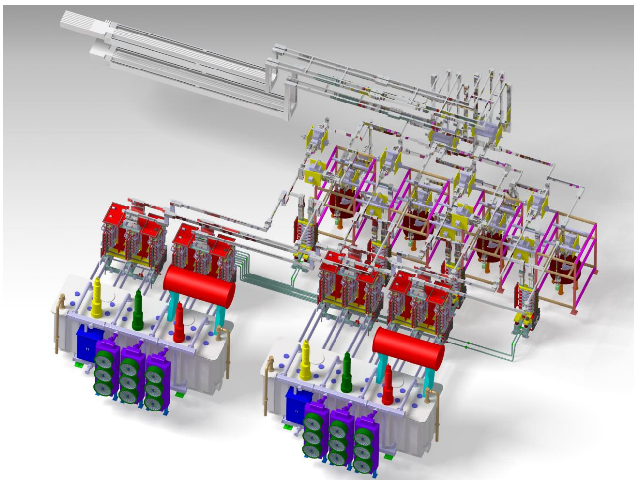
图 2 设备及母排连接图
