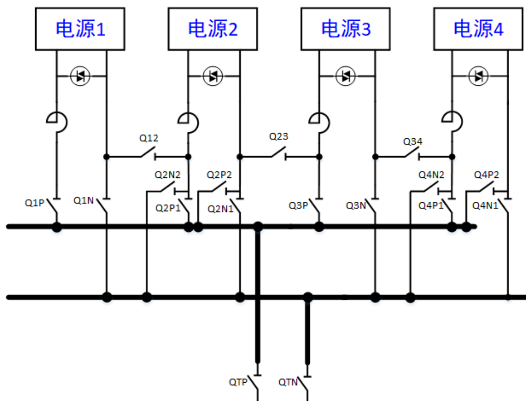
图 1 系统原理图
