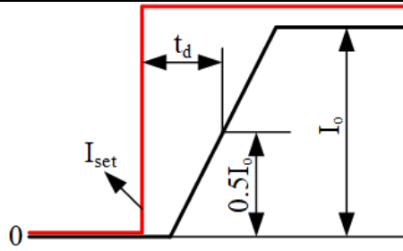
图 1 电流延迟示意图
