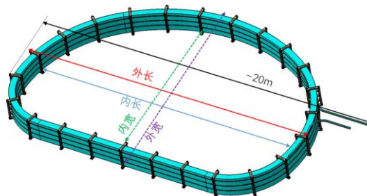
图 7. TF 中场线圈夹具分布示意图
