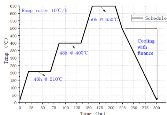
图 4. TF 高场线圈热处理制度
