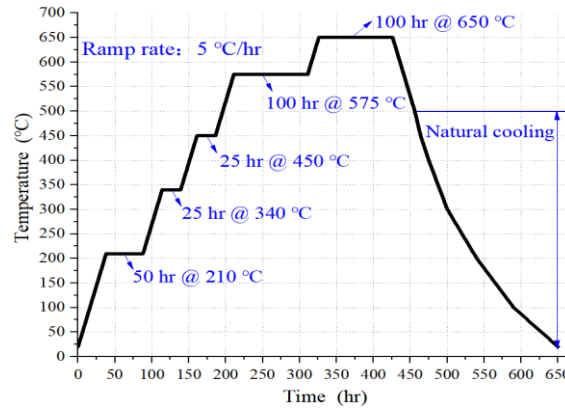
图 5. TF 中场线圈热处理制度
