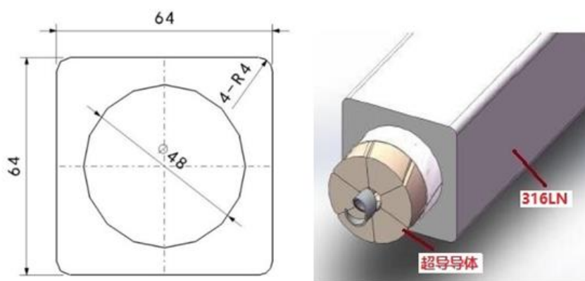
图 3. CRAFT TF 线圈导体截面及导体示意图
