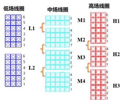
图 2. CRAFT TF 线圈组成截面图
