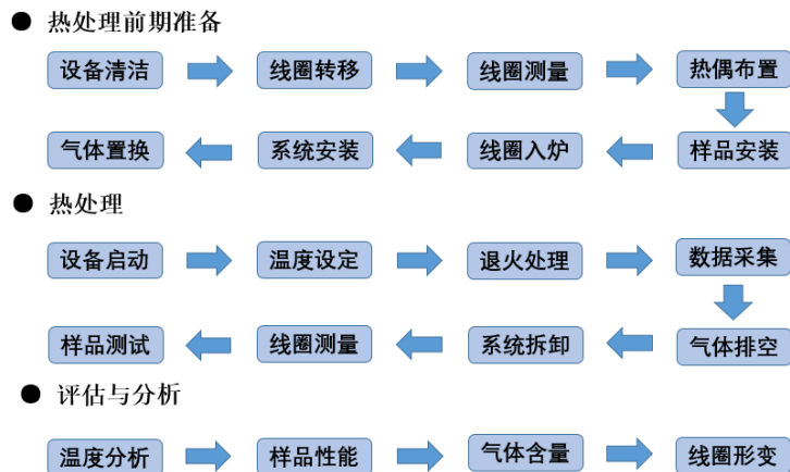
图 9. TF 线圈热处理过程工艺流程图
