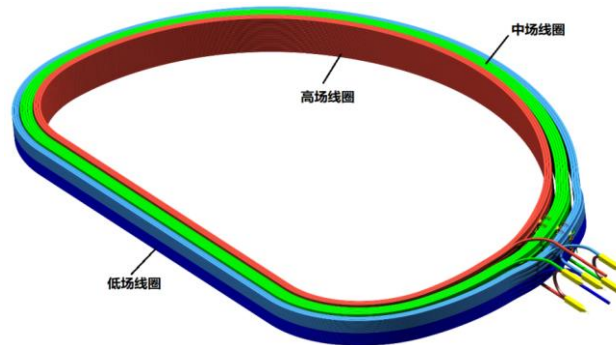
图 1. CRAFT TF 线圈示意图
