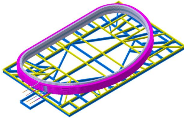
图 10. CRAFT TF 绕组热处理加强料盘示意图
