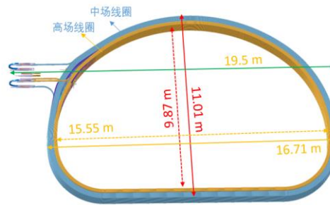
图 6. TF 高、中场线圈示意图
