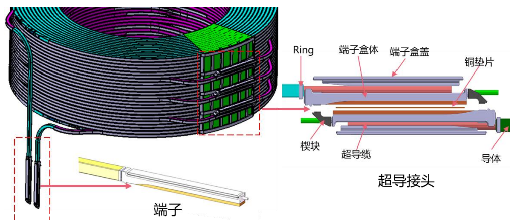
图 2 端子及接头示意图
