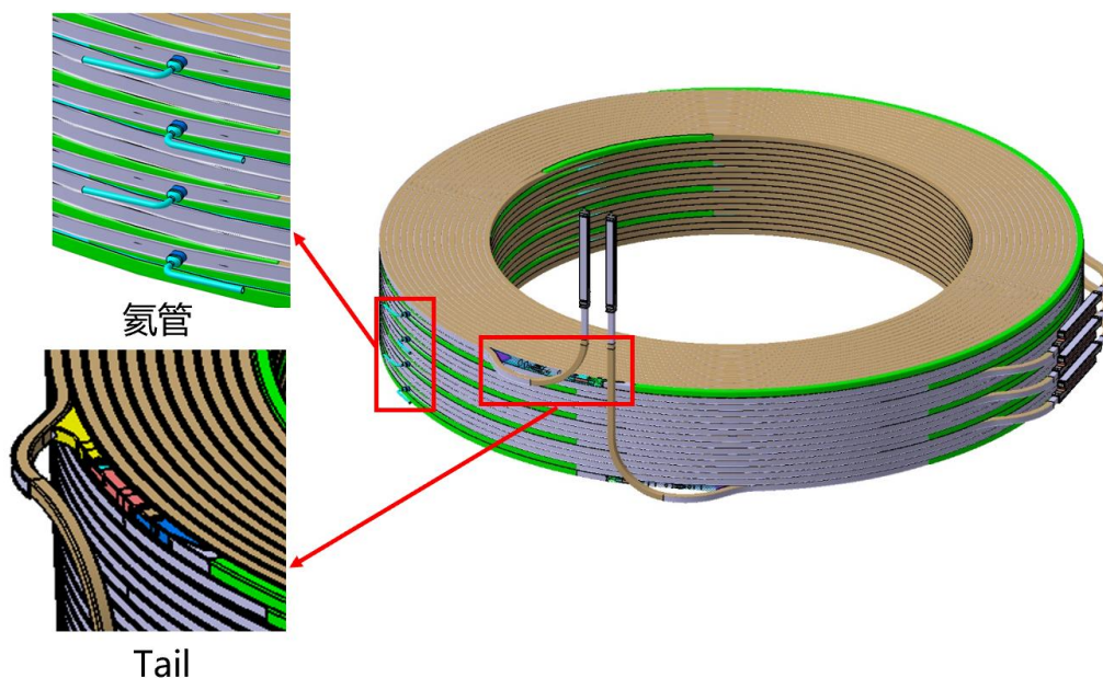
图 1 PF1 线圈示意图
