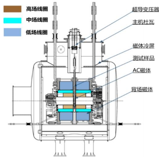
图 2 CRAFT 导体测试平台结构示意图
