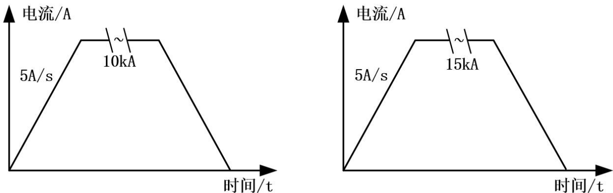
图 3 正常工作模式下的背场磁体电流波形
