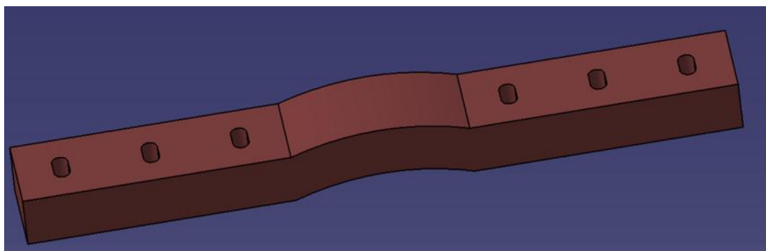
图 4 推荐单层铜母排形状 300 \times 50\text{mm} @ \phi 18\text{mm} \times 2
