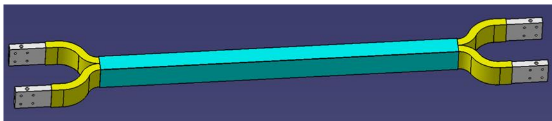
图 2 推荐铝叠层母排形状 200 \times 60\text{mm} \times 2 @ \phi 20\text{mm}
