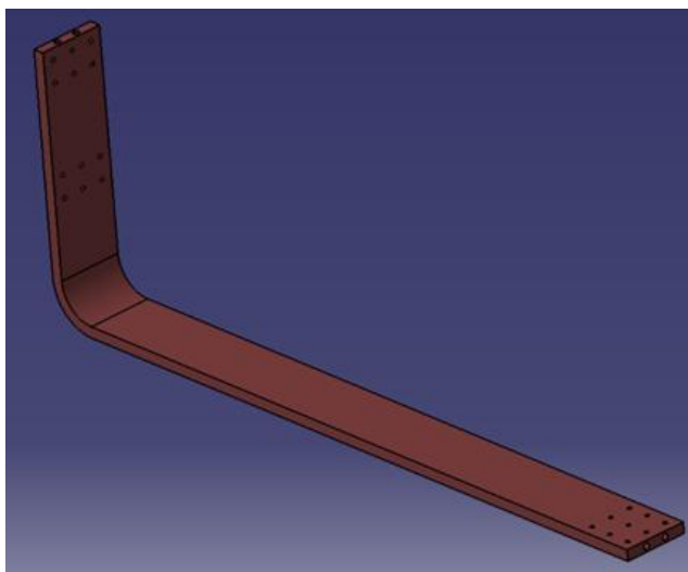
图 4 推荐单层铜母排形状 300 \times 50\text{mm} @ \phi 18\text{mm} \times 2
