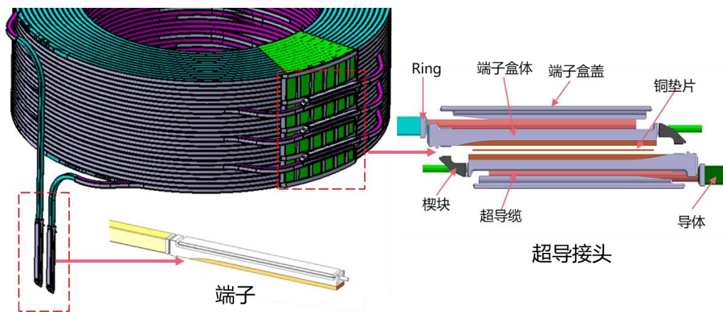
图 2 端子及接头示意图
