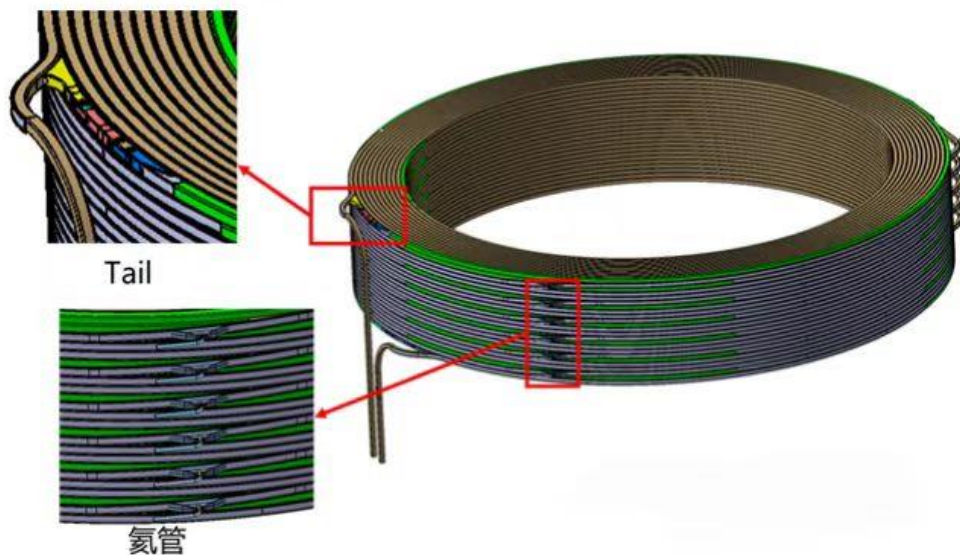
图 1 PF2 线圈示意图
