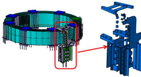
图 1 PF 磁体终端箱示意图
