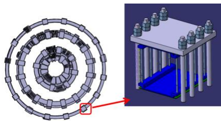
图 2 PF 磁体支撑夹具结构示意图
