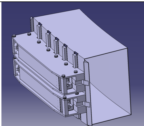
图 2 PF 接头夹具结构示意图
