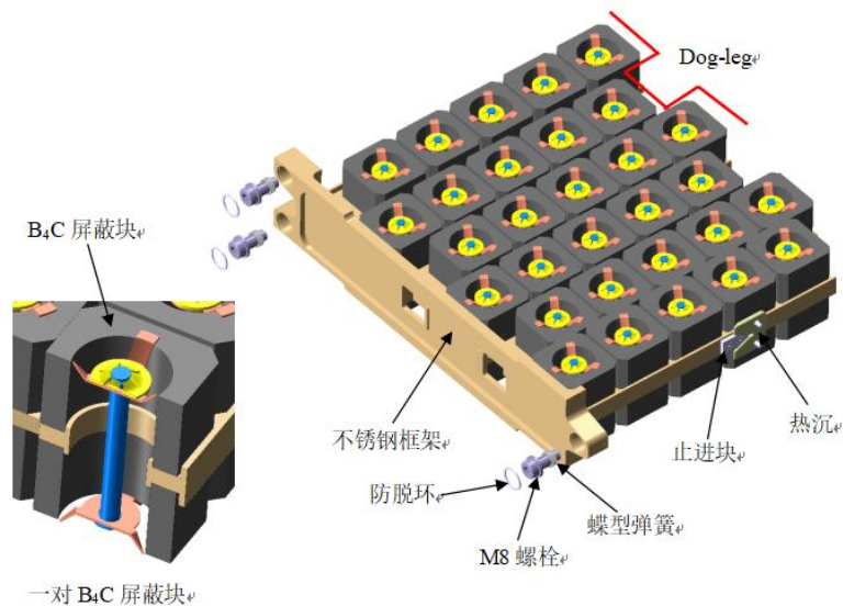
图 3-2 窗口插件结构组成
