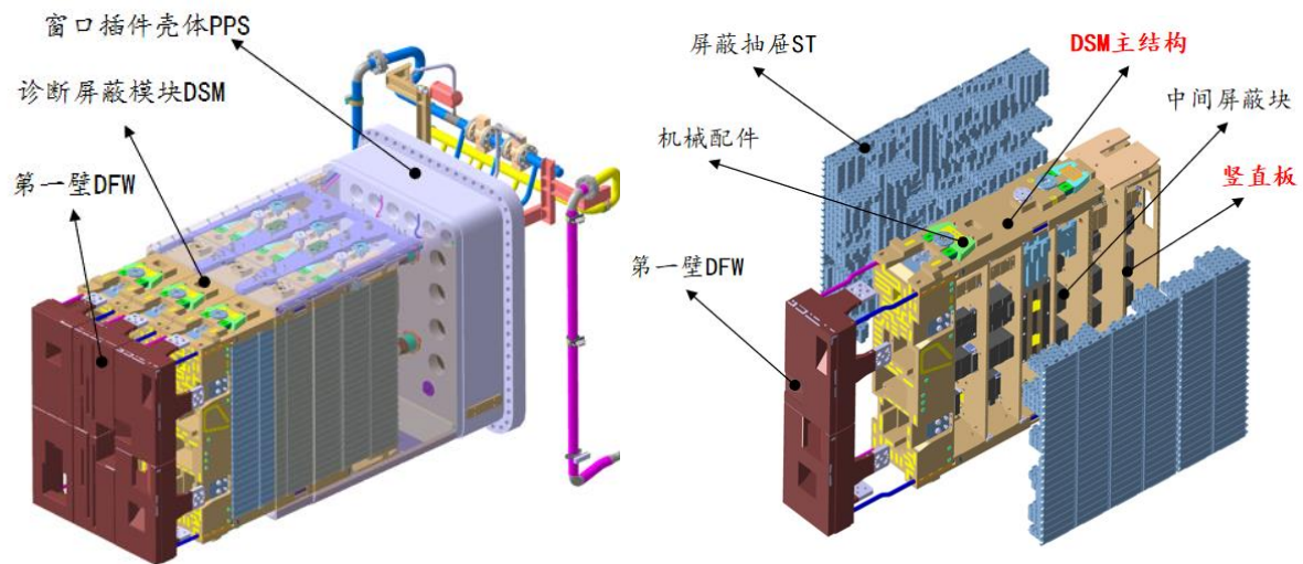
图 3-2 窗口插件结构组成
