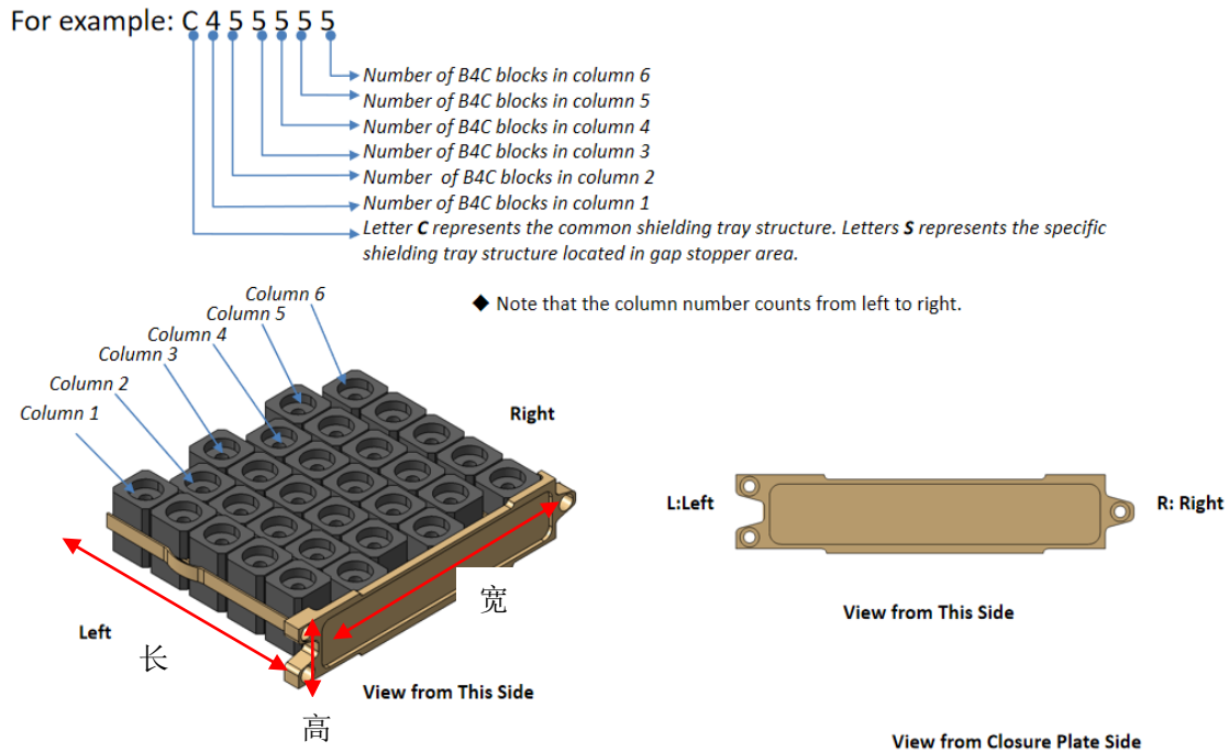
图 3-1 屏蔽托盘长度定义及标识规则
