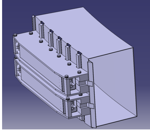
图 3 PF 接头夹具结构示意图
