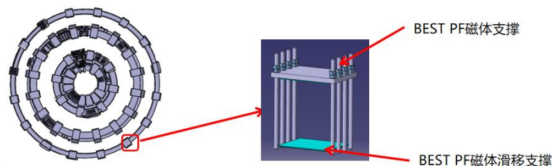
图 2 PF 磁体支撑夹具结构示意图
