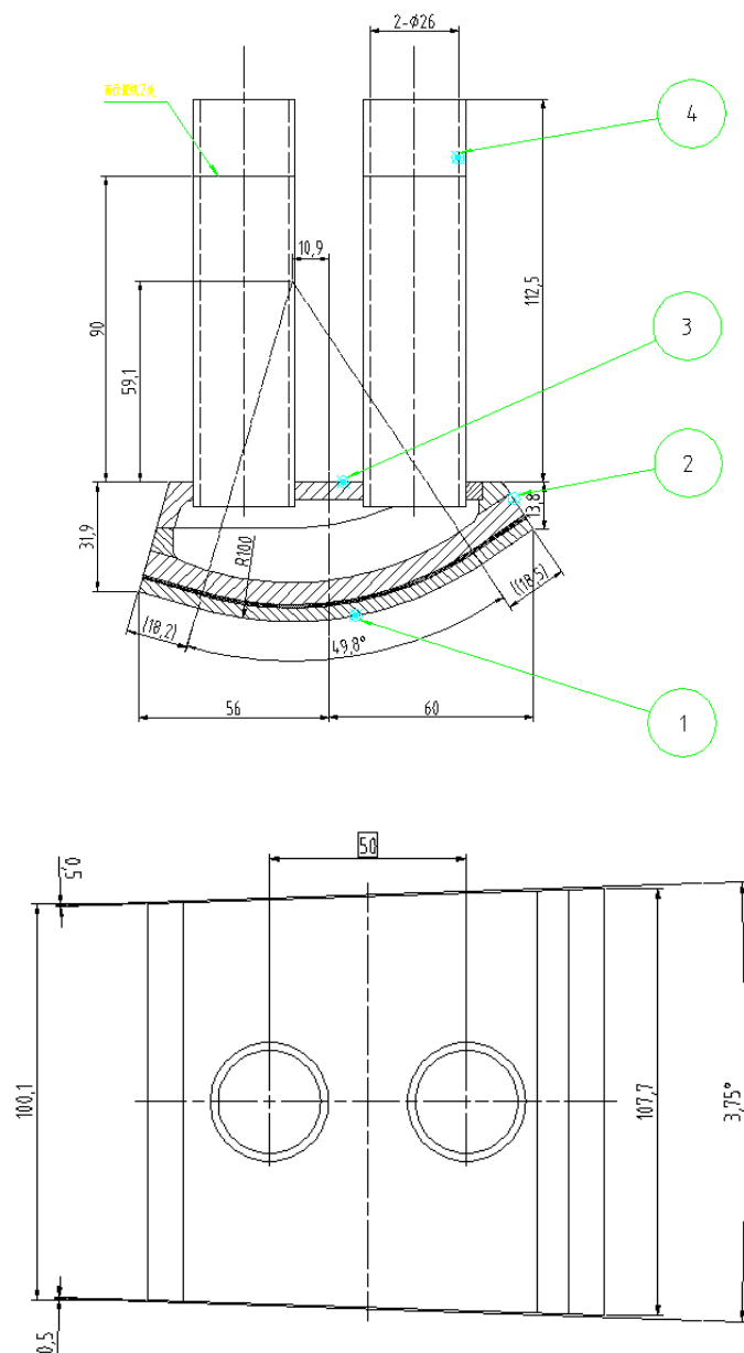
图 3 DOME 结构图
