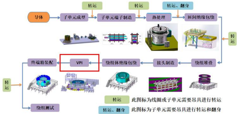
图 3 PF6 线圈制造流程
