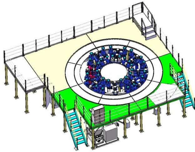
图 4 PF6 线圈 VPI 生产平台
