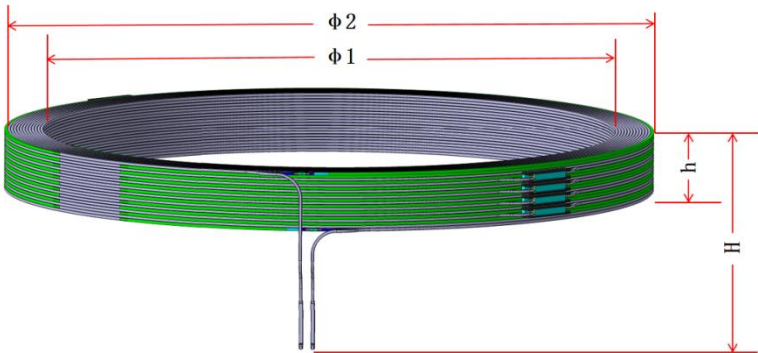
图 2 线圈主要尺寸示意图
