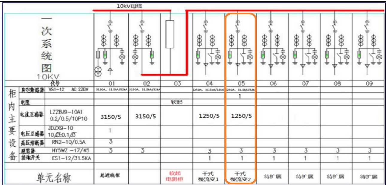
图 2.3.1.2 10kV 高压开关柜单线图
