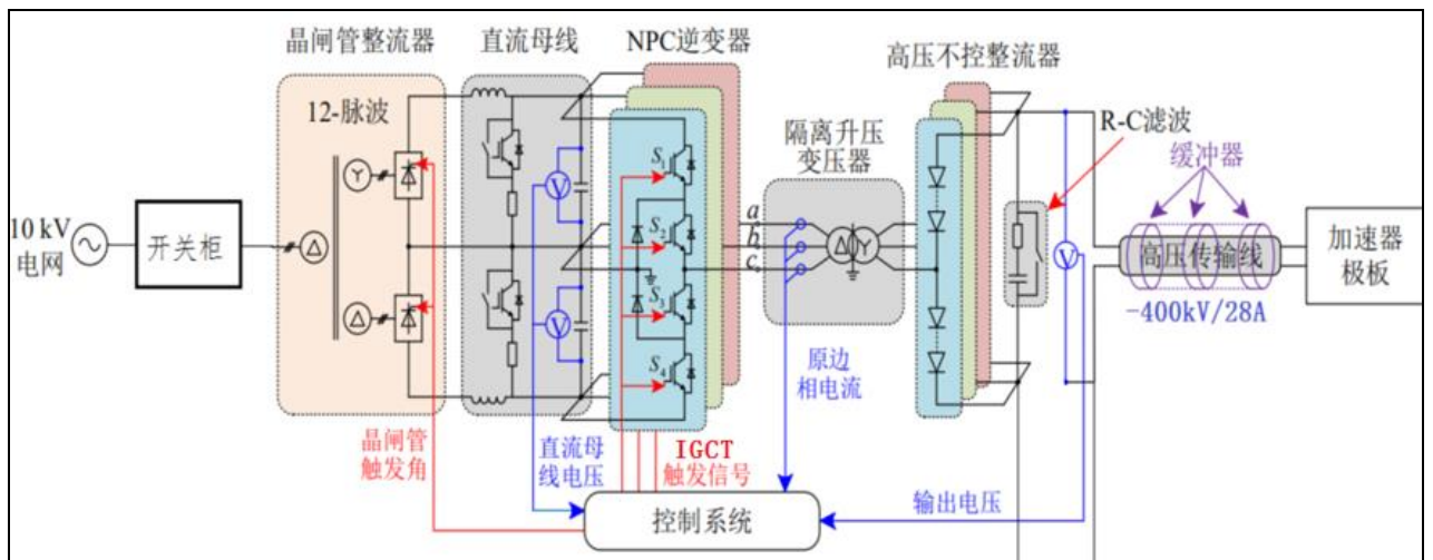
图 2.3.1.1 NNBI 高压电源拓扑结构图
