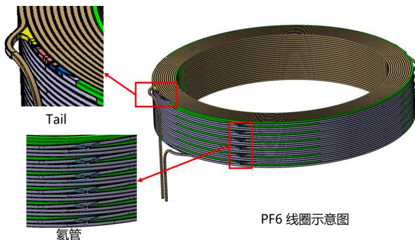
图 1 PF6 线圈示意图
