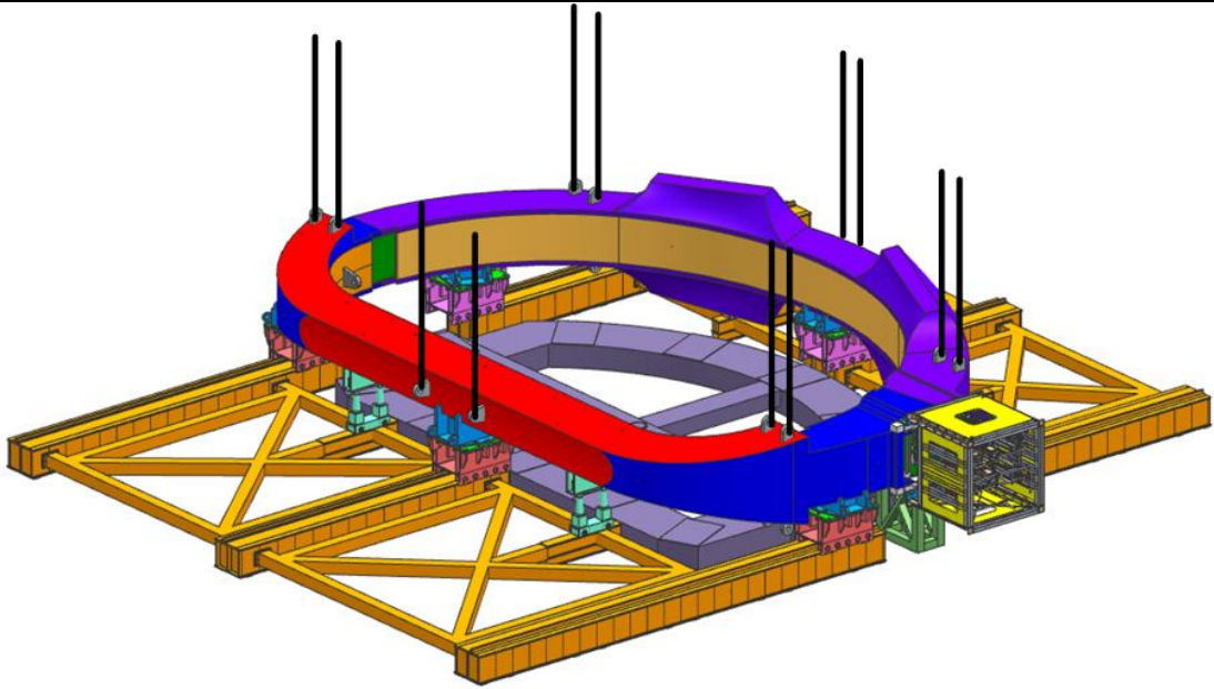
图 6 TF 磁体线圈盒
