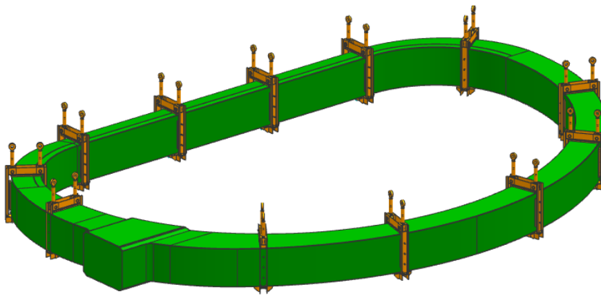
图 4 TF 绕组 12 个吊点形式示意
