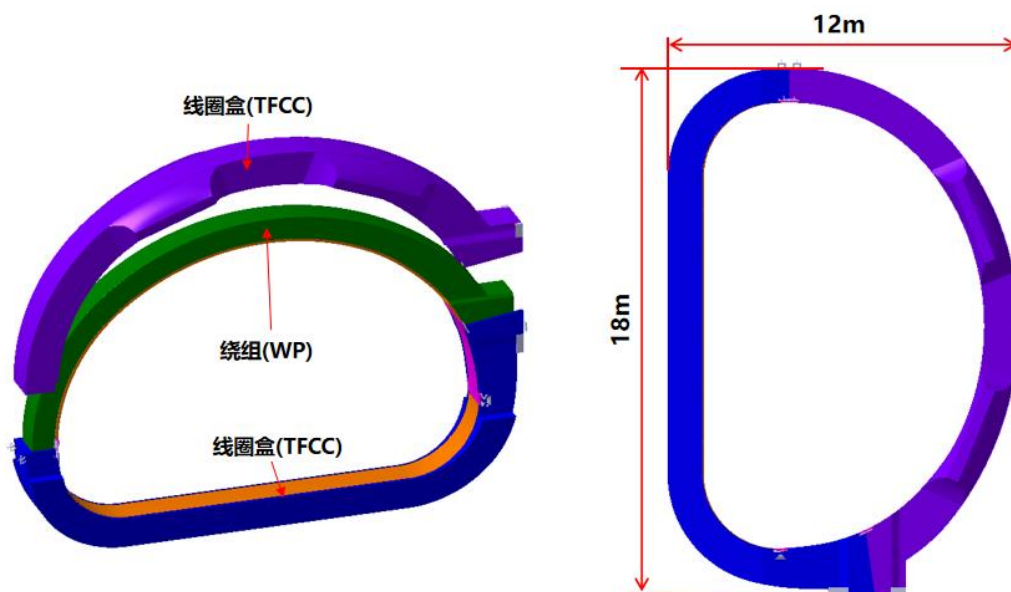
图 1. CRAFT TF 线圈主体结构
