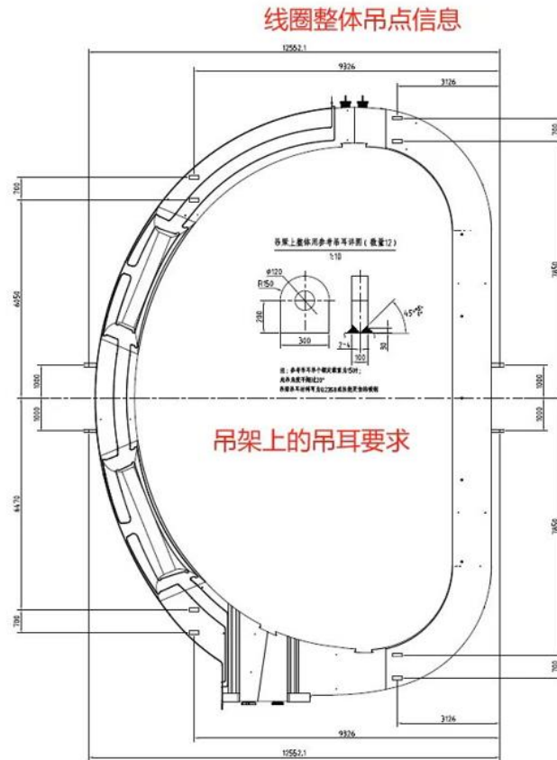
图 7 TF 磁体线圈盒
