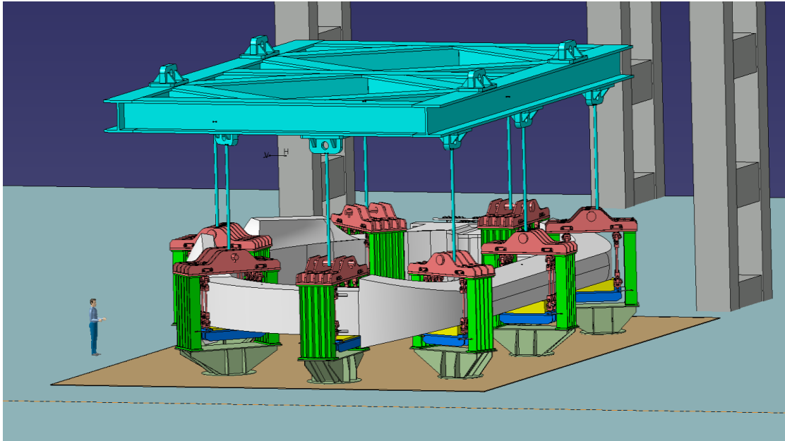
图 8 TF 磁体冷测试起吊形式
