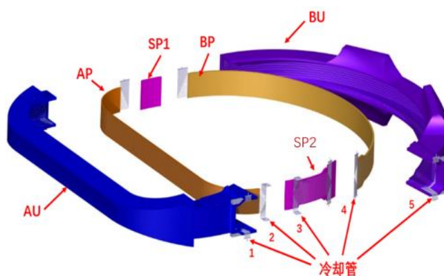
图 3 线圈盒部件结构
