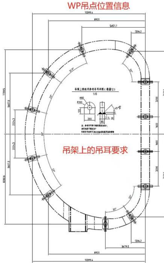
图5 TF 绕组吊点尺寸
