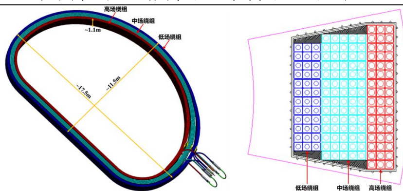
图 2.TF 线圈绕组(WP)结构图
