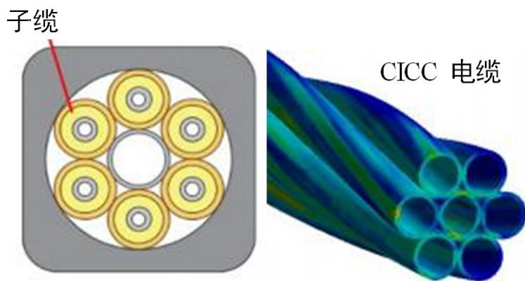
图1. 高温超导CICC 结构示意图
