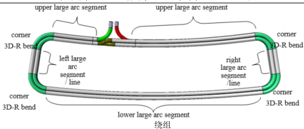
图 1-2 UP-ELM 线圈
