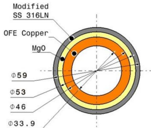
图 1-1 SSMIC 导体
