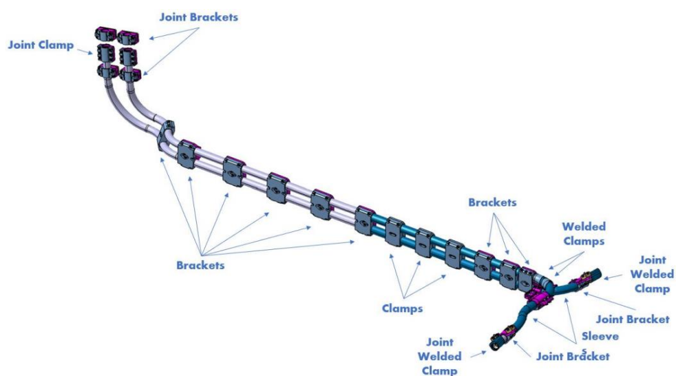
图 1-3 UP-VS Feeder
