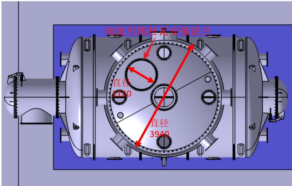
图 1 电流引线杜瓦于主机系统杜瓦对接接口
