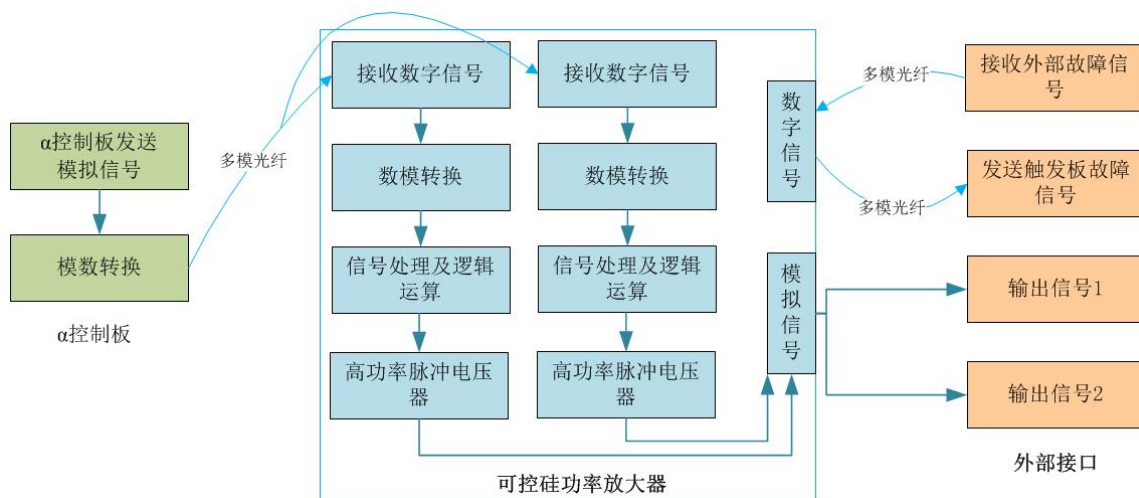
图 1 可控硅功率放大器控制板设计技术方案
