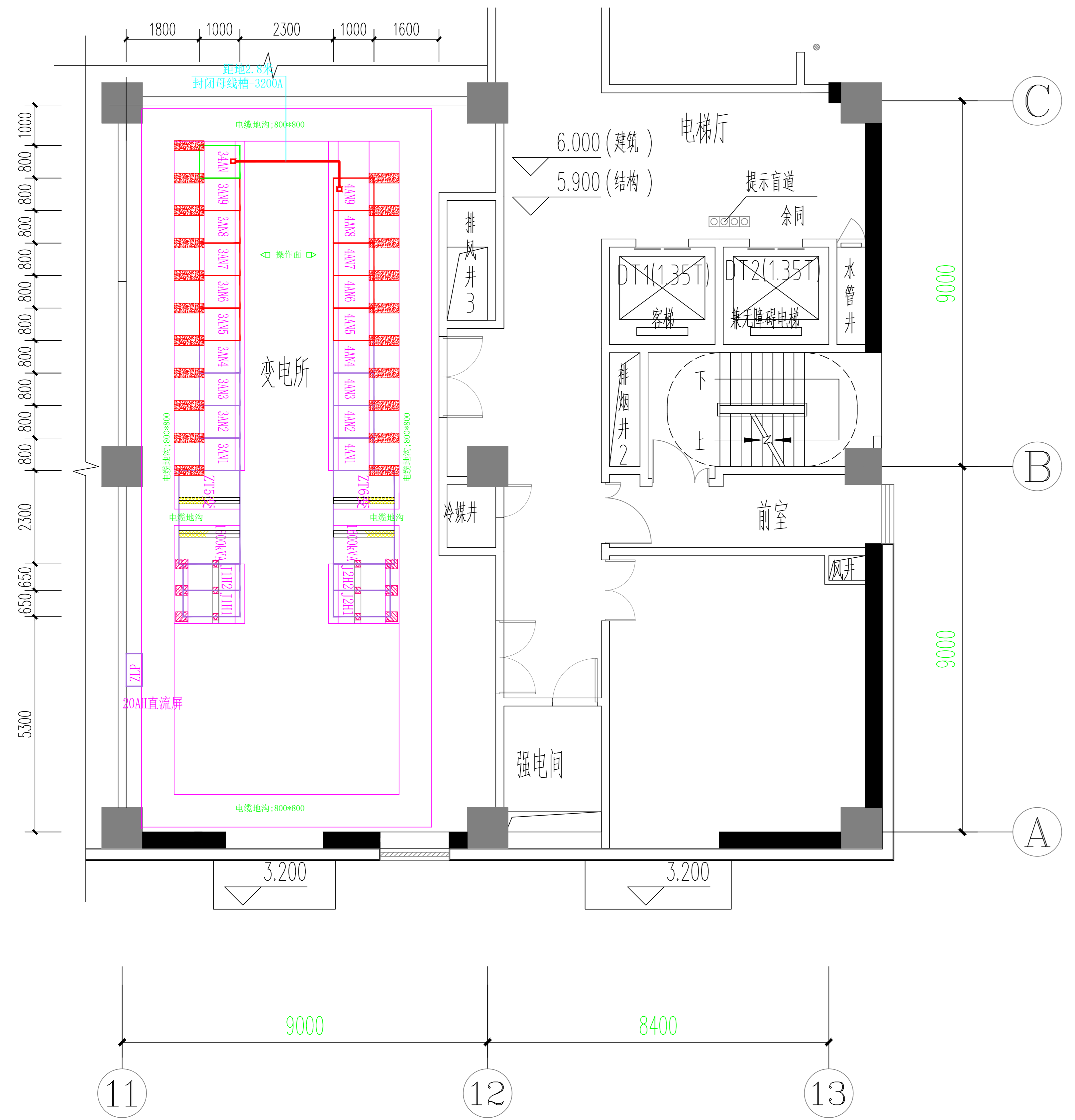
夹层变电所布置平面图
