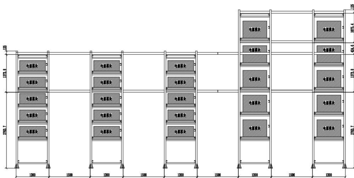
图 1 电源模块支架
