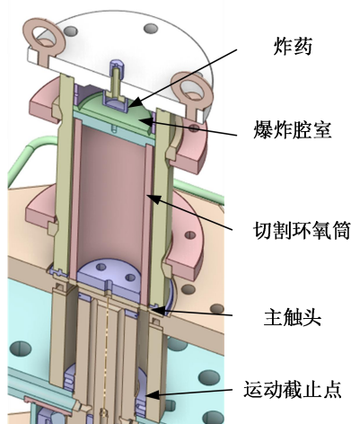
图 1 爆炸开关切割环氧筒和主触头示意图
