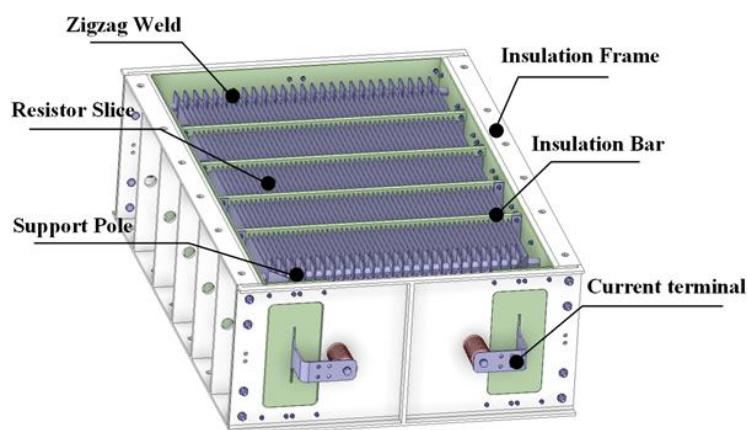
图 1 电阻模块
