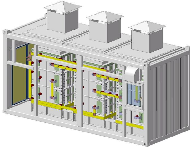
图 3 电阻堆栈安装示意图
