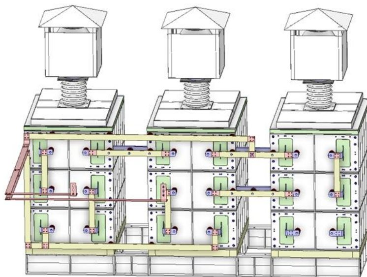
图 2 8 模块连接示意图
